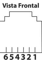
Conector Hembra RJ-11 Del PumpMonitor/FaseAlert
