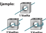
Numero de vueltas del cable de alimentación en el Transformador de corriente para menos de 6 Amp.
